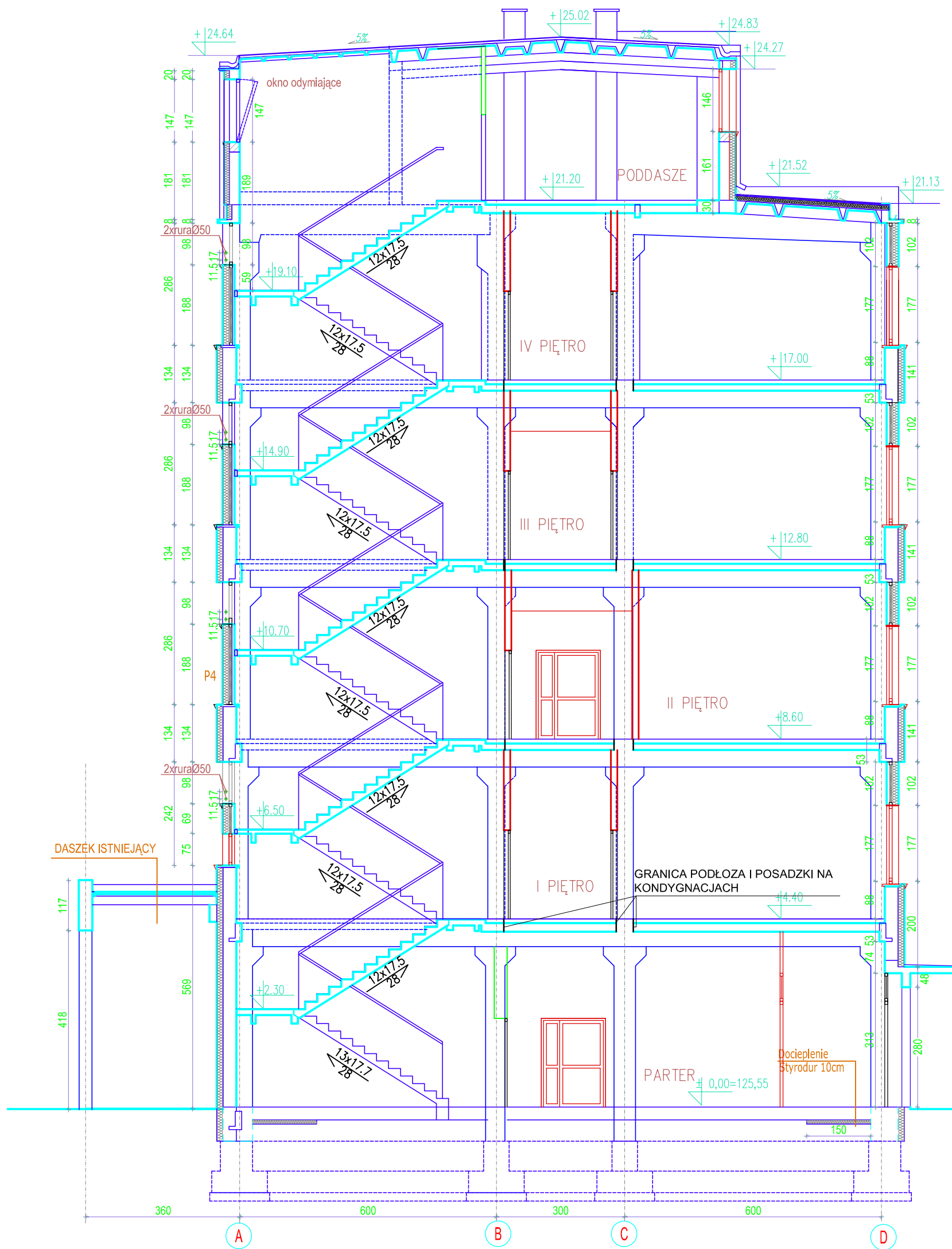
PRZEKRÓJ II-II
