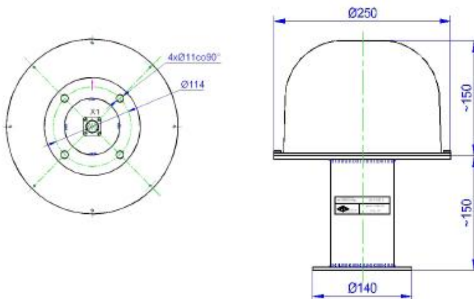
Głowica antenowa
